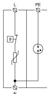
Vnútorňá schéma zapojenia
